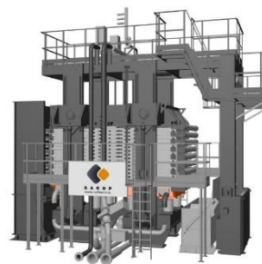
Башенный фильтр пресс
