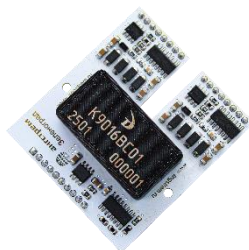
Двухканальное ядро драйвера IGBT
