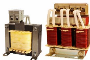
PCO и PCT сетевые дроссели
