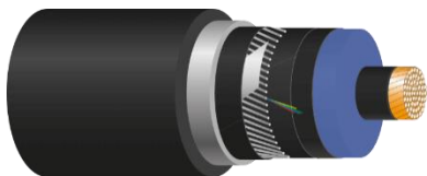
Силовой кабель 60-220 кВ с изоляцией из сшитого полиэтилена
