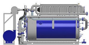
Водогрейный котел МЦПТК
