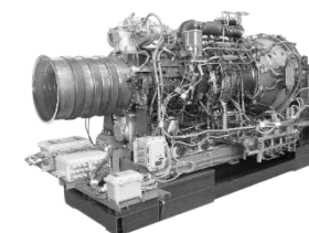
Морской газотурбинный двигатель E70/8RD
