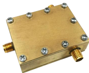
Синфазный делитель/сумматор мощности на 2 РК-СДМ-2-1,5/18
