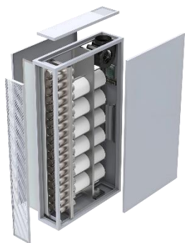
Напольный рециркулятор Аэролайф А-1000
