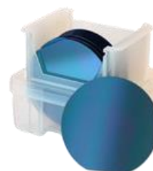
Кремниевые эпитаксиальные структуры
