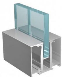
Зажимной комплект в стиле Лофт с применением профиля направляющей М1 ФСТ-146
