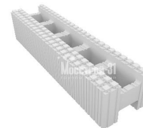
Несъемная опалубка серия 30
