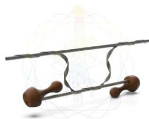
Гаситель ветровых колебаний универсальный ГВКУ- 10,4/10,9-2,4/1,6-450-11,0-01- 2-ТРИАС
