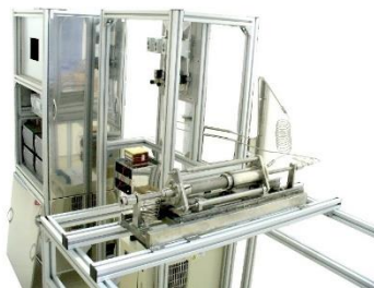
Лабораторная установка для нанесения покрытий с помощью газотранспортных реакций на экспериментальные образцы деталей сложной формы
