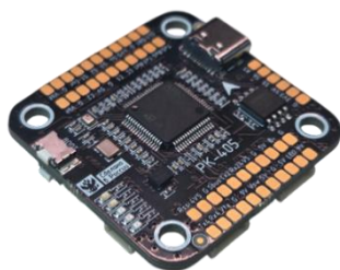
Полётный контроллер РК-405 3-поколение
