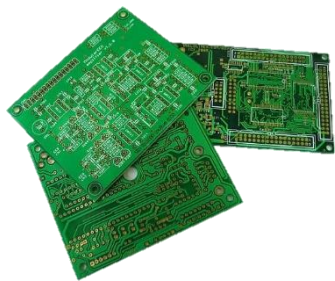
Печатные платы односторонние, двусторонние, многослойные
