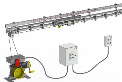
Механизм дороги занавеса раздвижной прямой ПМЗ с электроприводом
