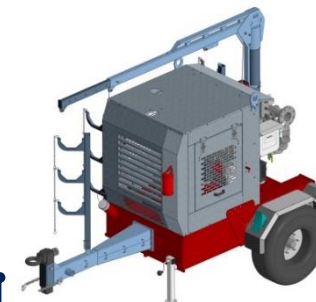
Насосная станция DNS.SHP-2 T512/T712
