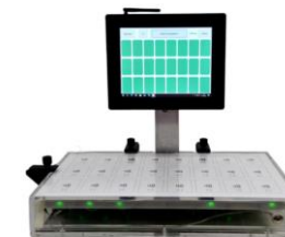
Устройство для тестирования инлеev и программирования карт в листах v.2.0
