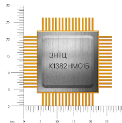
СБИС магнитного энкодера положения K1382HM015
