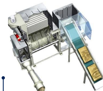
Автоматические системы растаривания
