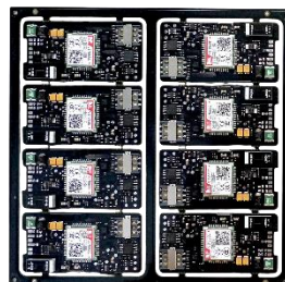
Плата с двухсторонним монтажом
