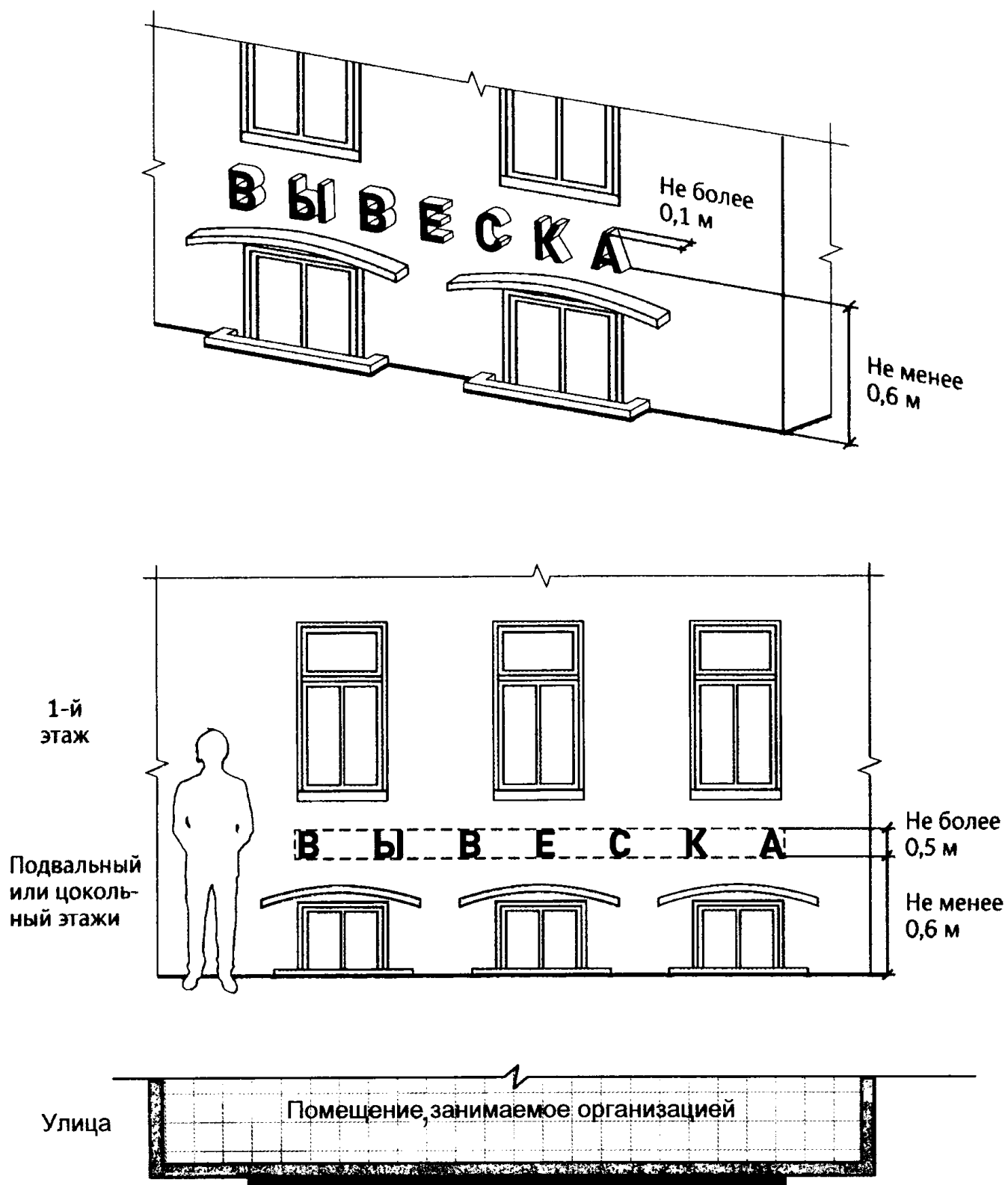
3.5.2. Размещение информационных конструкций (вывесок) на подложке.
